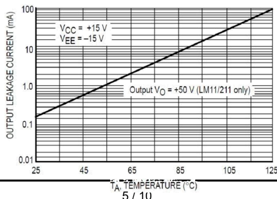
输出漏电流与温度关系
