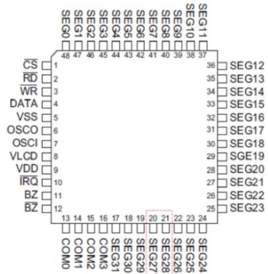
HT1621B 48LQFP-A
