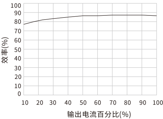
效率Vs输出负载（标称输入） R-78Exx-0.5
