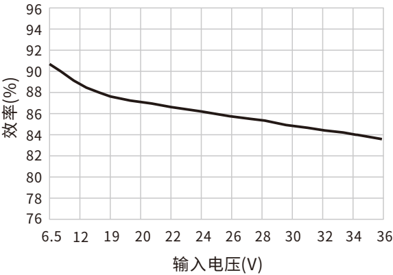
效率Vs输入电压（满载） R-78Exx-0.5
