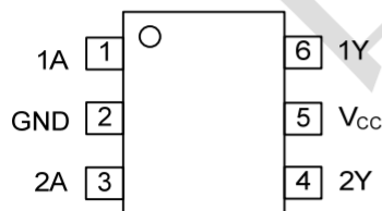
SOT23-6/SOT363
