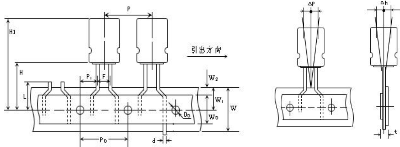
Taping Table
