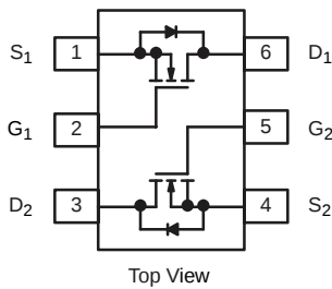
SOT-363 SC-70
