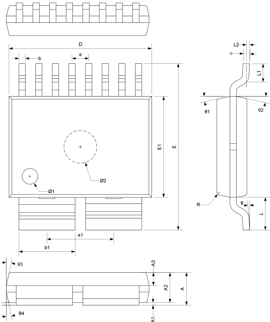
SOW10 封装
