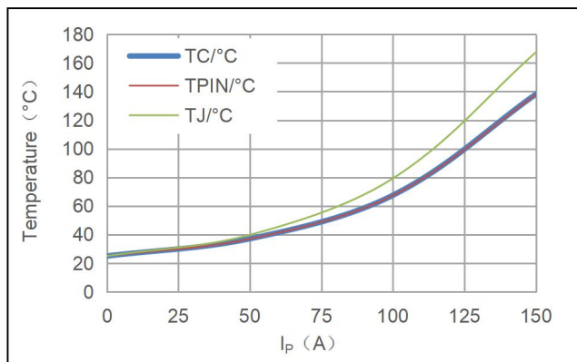
芯片温度 T_C & 引脚温度 T_{PIN} & 芯片结温 T_J vs 原边电流 I_P
