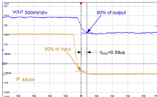
V OUT 下降阶跃响应波形图
