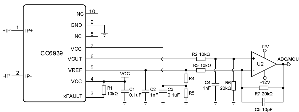
零点迁移应用（基准输出模式）
