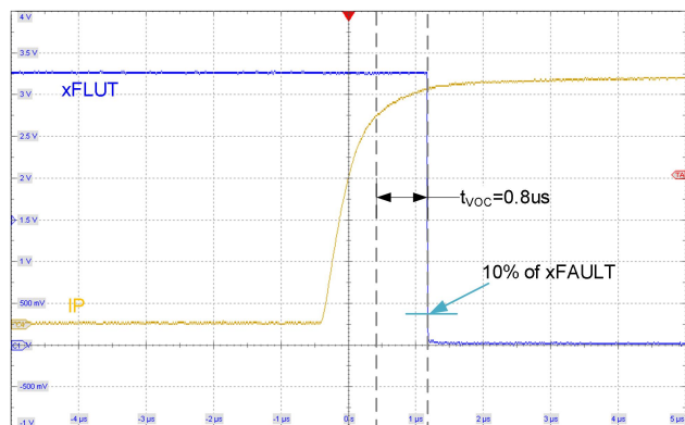
xFAULT 响应 t_{voc} 波形
