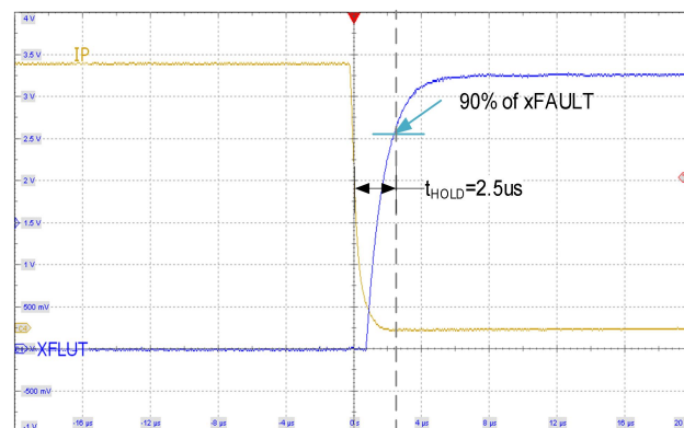
xFAULT 响应 t_{hold} 波形
