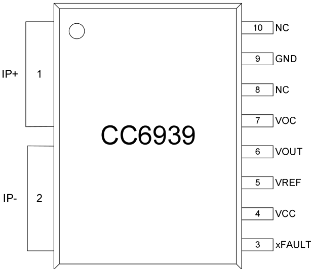
SOW10 封装
