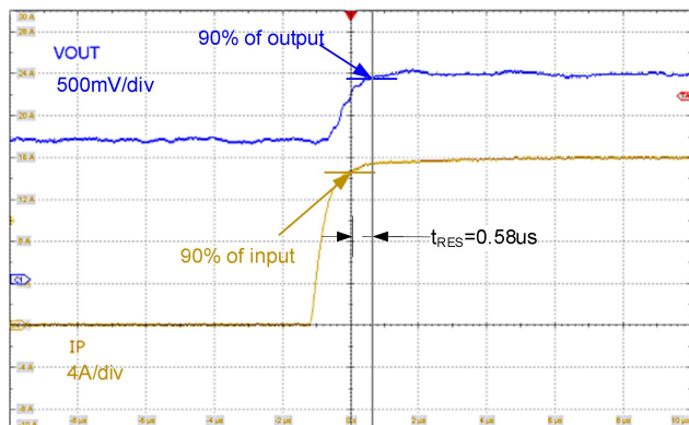
V OUT 上升阶跃响应波形图
