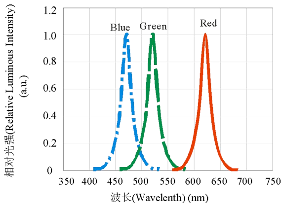
光谱分布特性曲线 Relative Spectral Distribution
