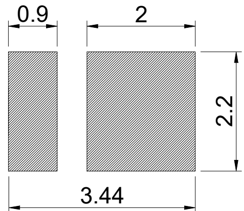
焊盘建议图
