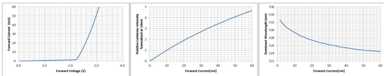
I-V 曲线
