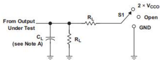
图3 负载电路
