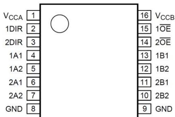
图 2 引脚排列图（顶视图）
