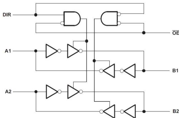
图 1 功能框图
