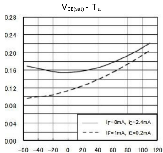
图 10：饱和电压 VS 温度
