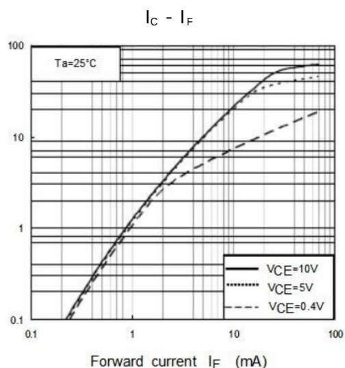
图 7：集电极电流 VS 正向电流
