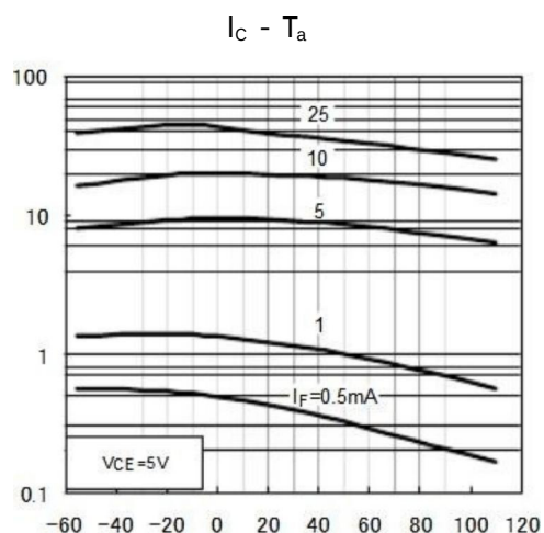
图 12：集电极电流 VS 温度
