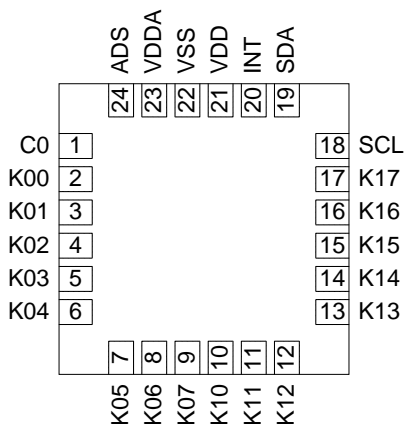
QFN24 引脚图
