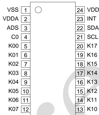
SSOP24 引脚图
