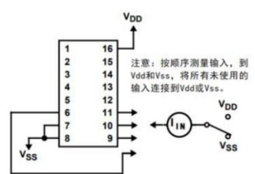
Fig.4 输入电流
