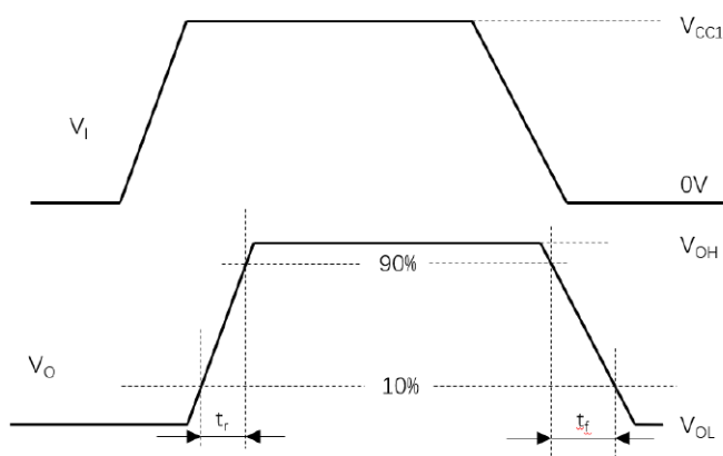
图 6 . 传输时间波形测量
