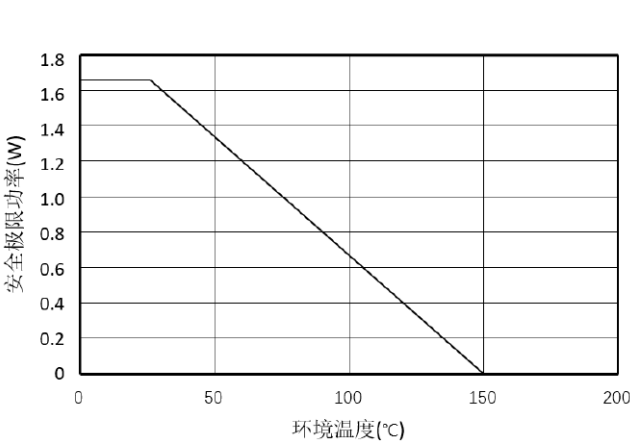
图 3.热降额曲线, 依据 DIN V VDE V 0884-10 的安全限值与环境温度的关系
