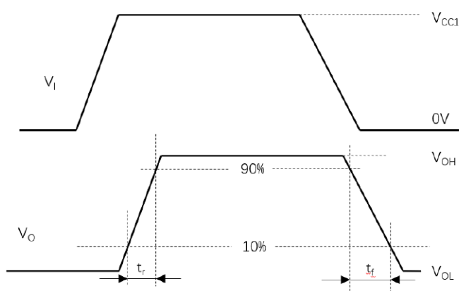
图 6 . 传输时间波形测量
