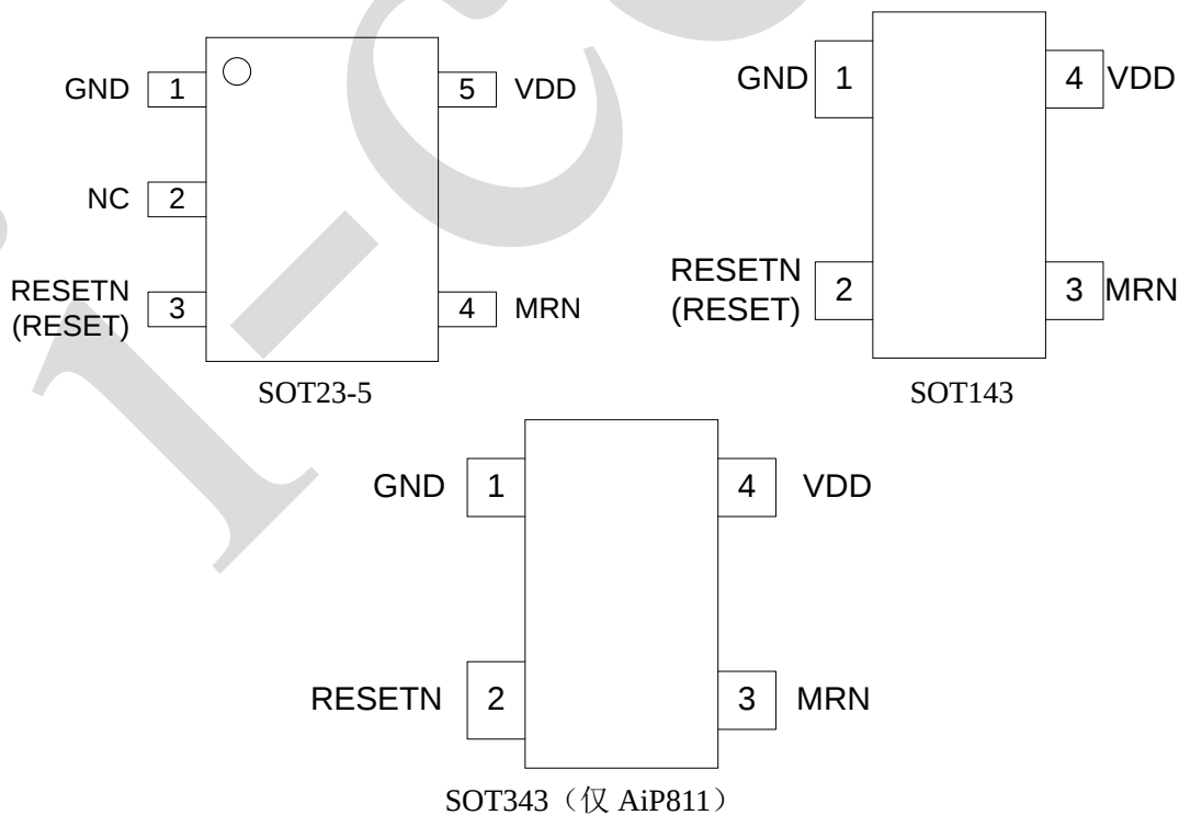
图 2、引脚图
