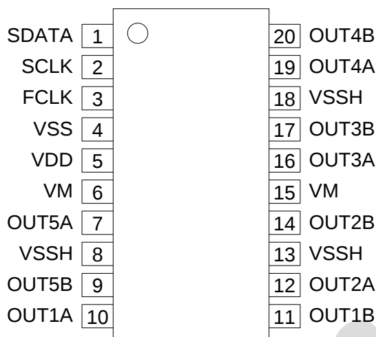
图 2 TSSOP20 封装引脚图
