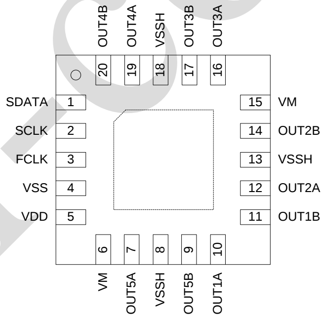
图 1 QFN20 封装引脚图
