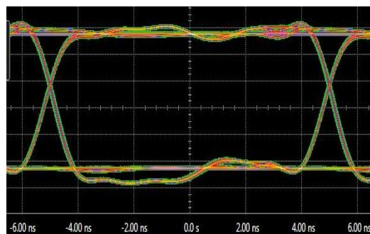
图 8. 眼图
