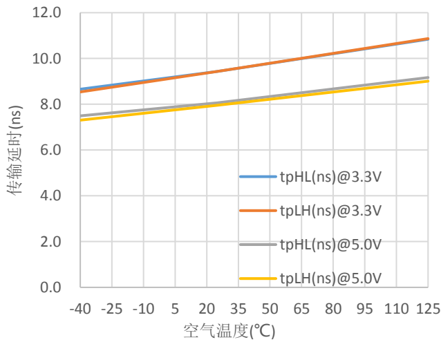
图 4. 传输延时 vs. 空气温度
