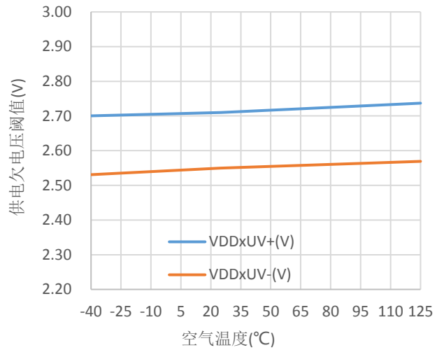
图 4.UVLO vs. 空气温度
