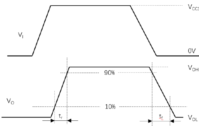
图 5. 传输时间波形测量
