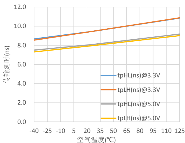
图 6 . 传输延时 vs. 空气温度
