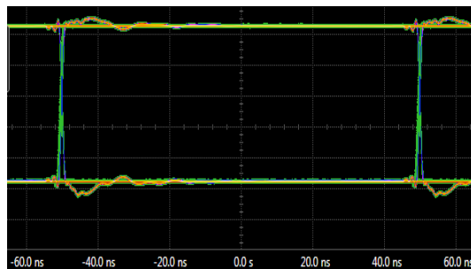
图 10.眼图
