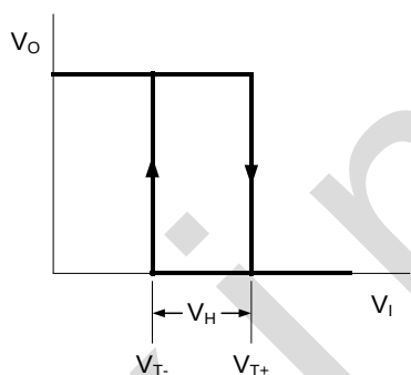
图6 传输特性
