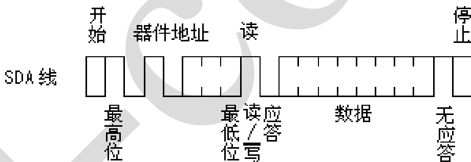
图 10、当前地址读操作
