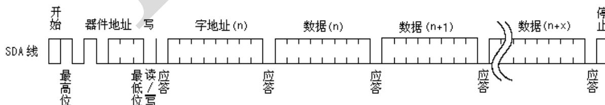
图 9、页写
