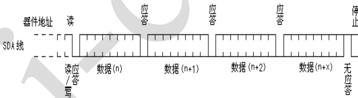
图 12、顺序地址读操作
