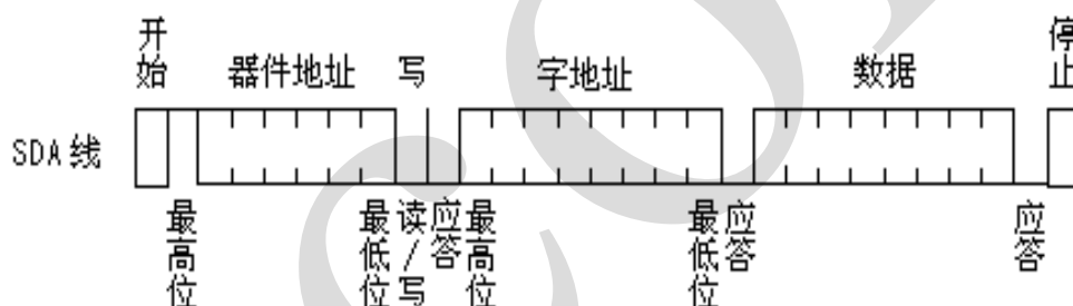
图 8、字节写
