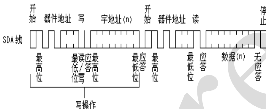
图 11、随机地址读操作
