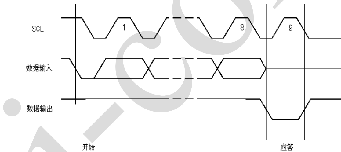
图 7、输出响应
