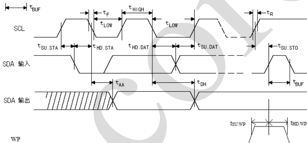
图 5、总线时序
