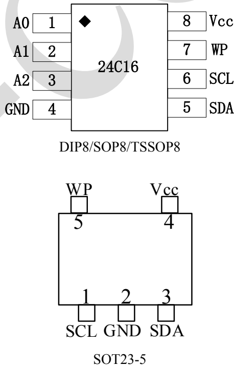
图 2、引脚排列图
