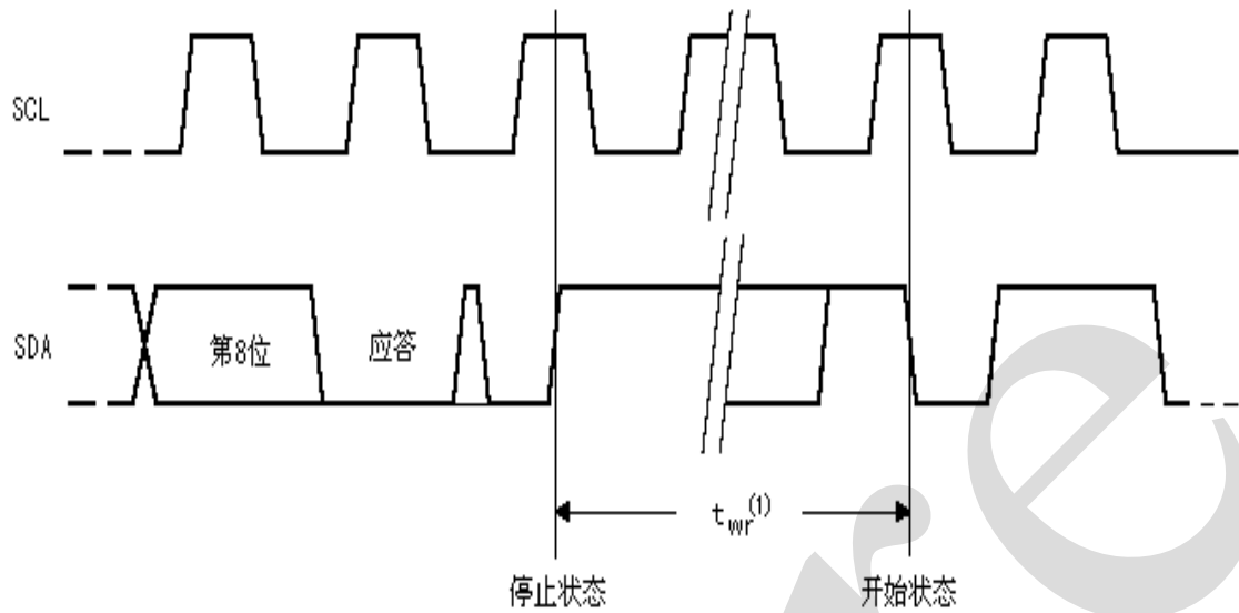
图 6、写周期时序
