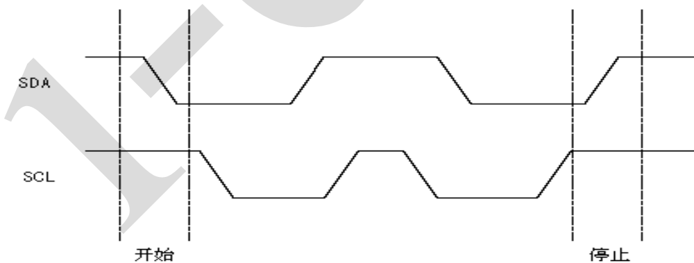
图 4、开始、停止时序图
