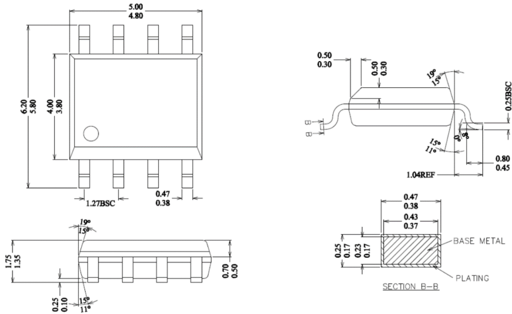
图 10. SOP-8 封装外形尺寸-尺寸单位(mm)
