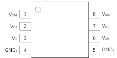
图 2. 管脚定义
