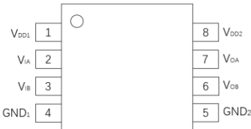
图 3. 管脚定义
