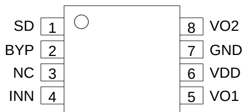
图 1、引脚排列
