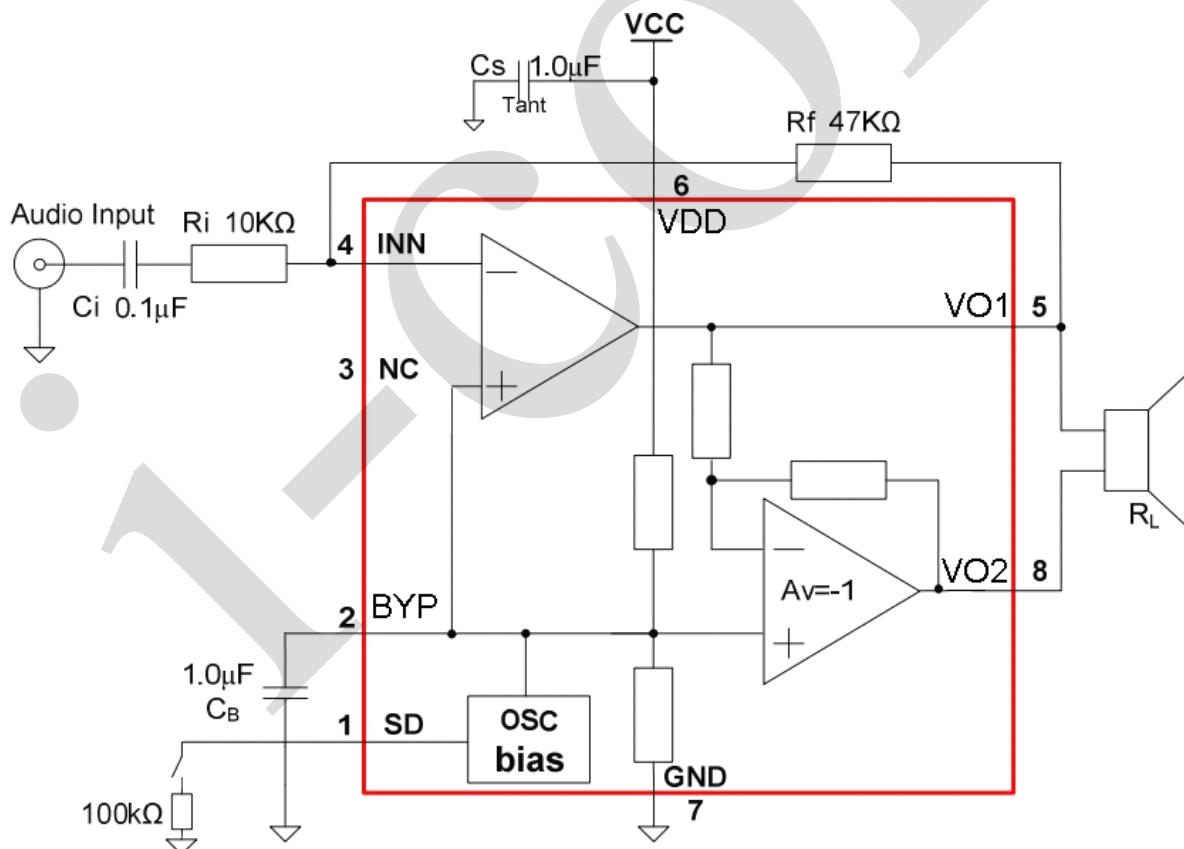
图 2、AiP4890D 典型应用图
