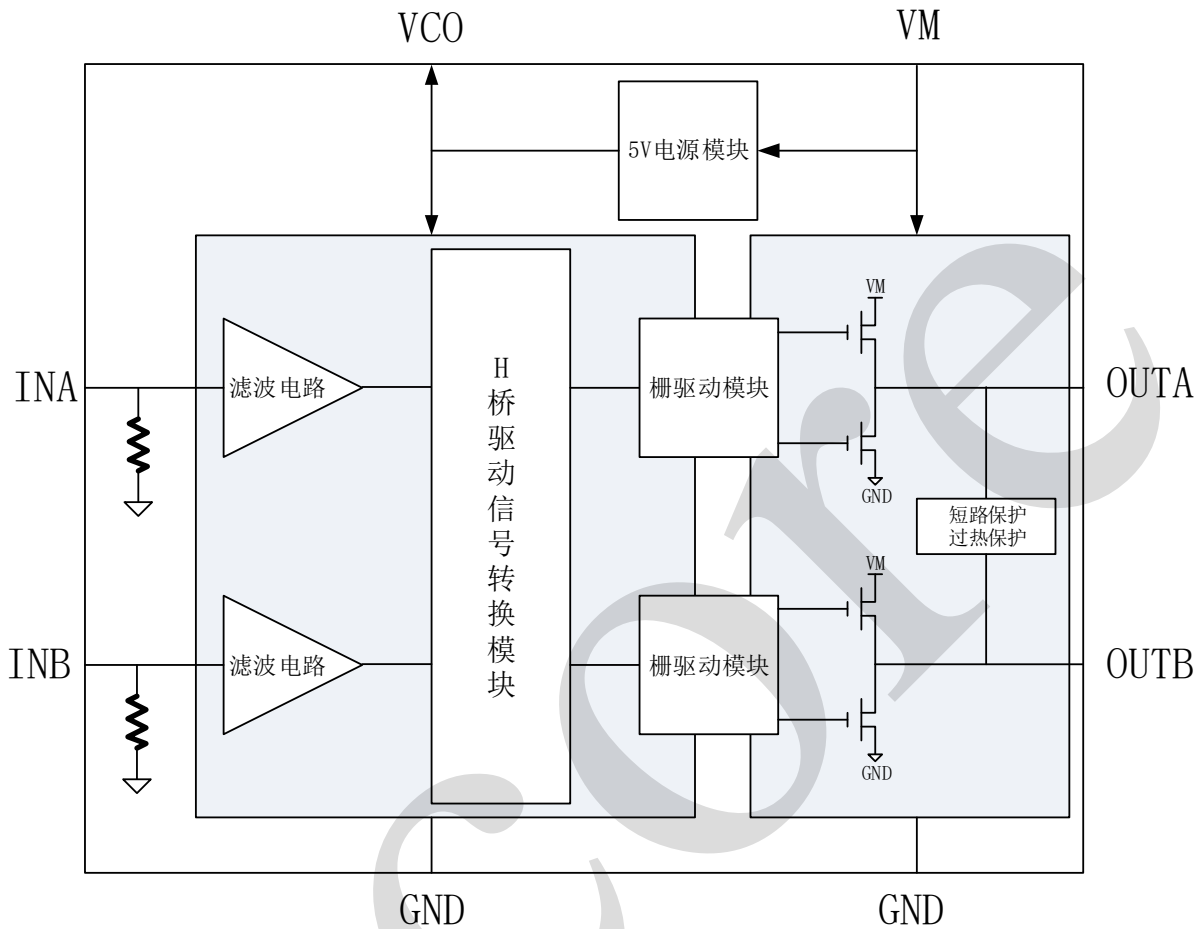
图 1、功能框图
