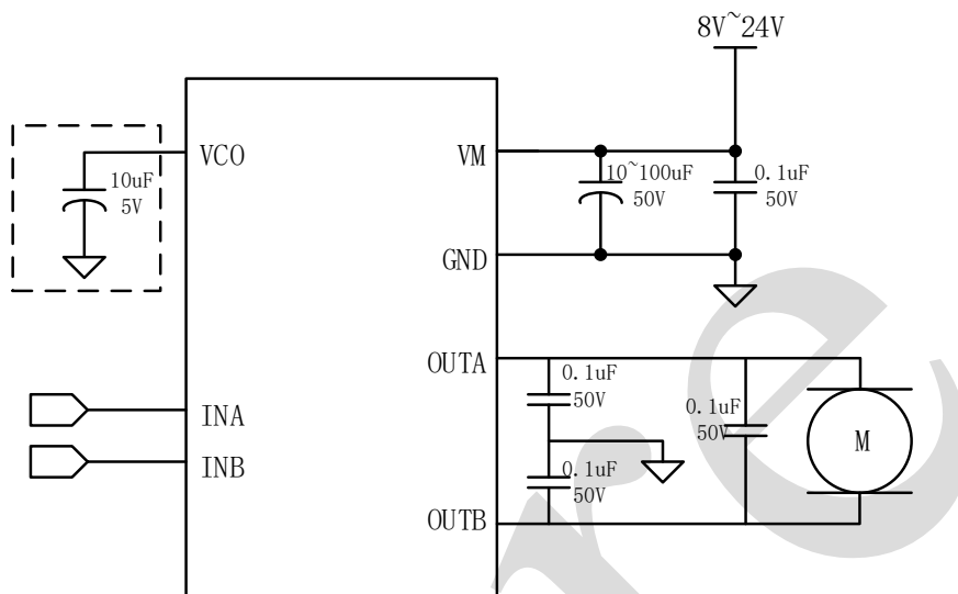
图 4、典型应用图
