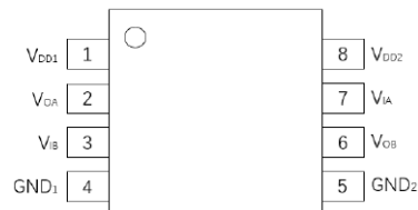
图 2. 管脚定义
