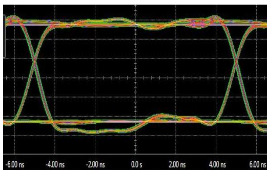
图 8. 眼图
