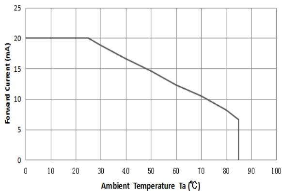
最大正向电流与环境温度特性曲线
