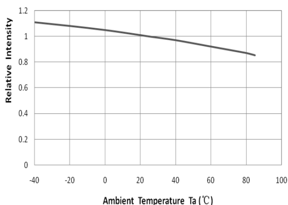
相对光强与环境温度特性曲线
