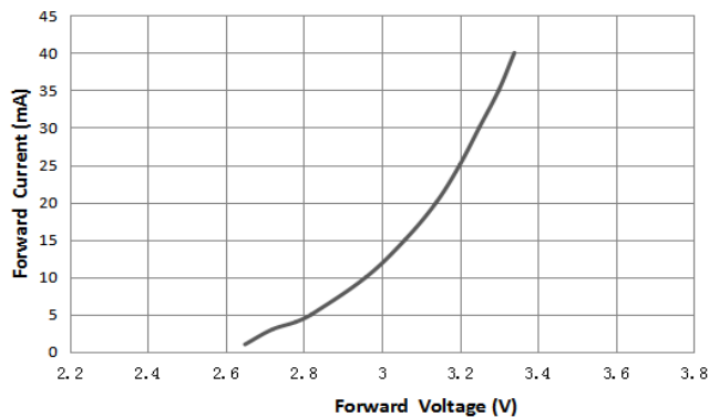
伏安特性曲线
