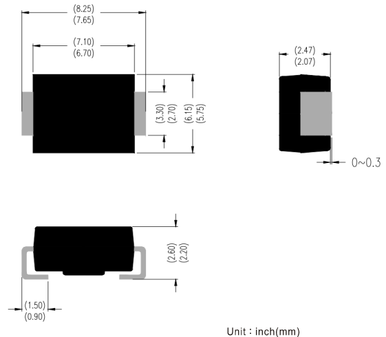
DO-214AB (SMC)
