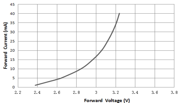
伏安特性曲线
