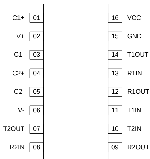
SOP -16 PKG
