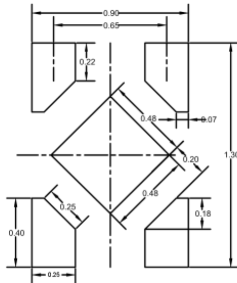
Detail A: (PIN1 shape)
