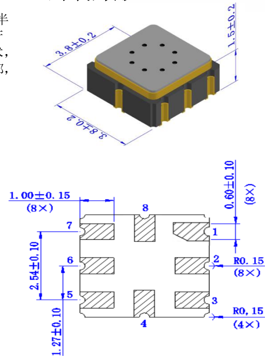
底视尺寸图(单位: mm)
