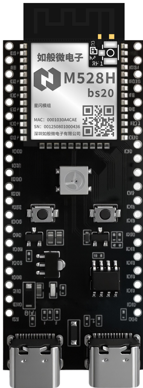
图 3: E528H-BS20 正面
