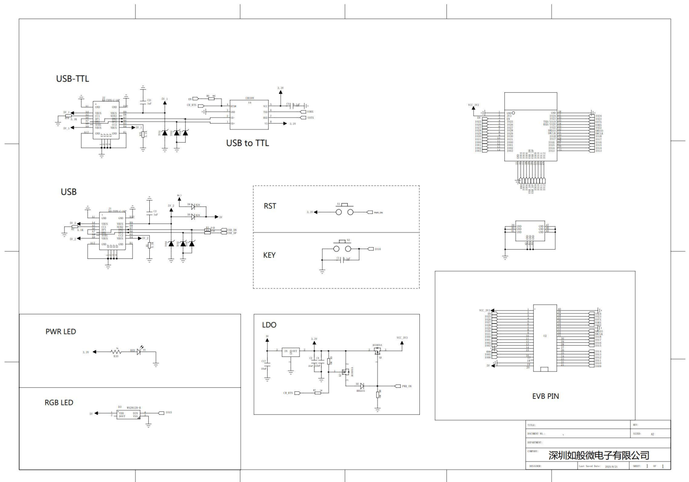
图 6: E528H-BS20 开发板原理图
