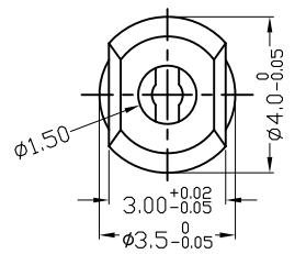
轴心部尺寸详图 2:1
