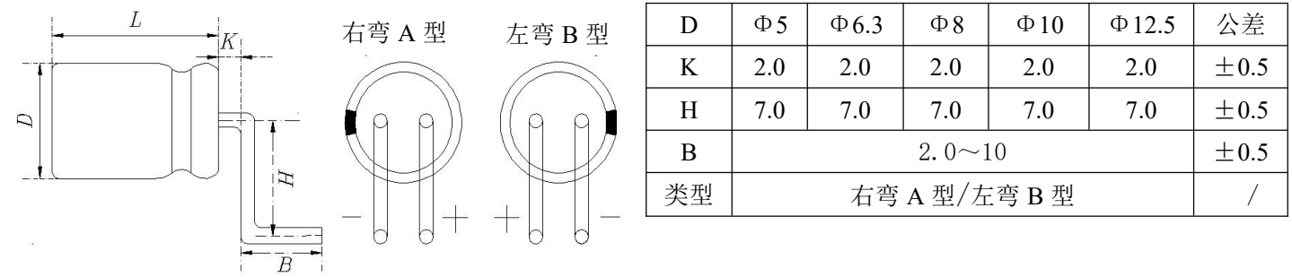
编带外型尺寸 A 图
