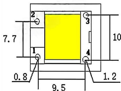
底视图
