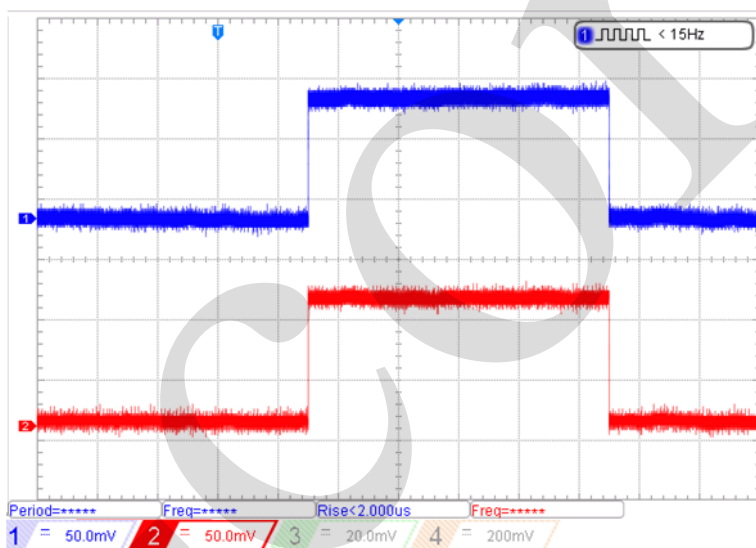
图 3 小信号响应
