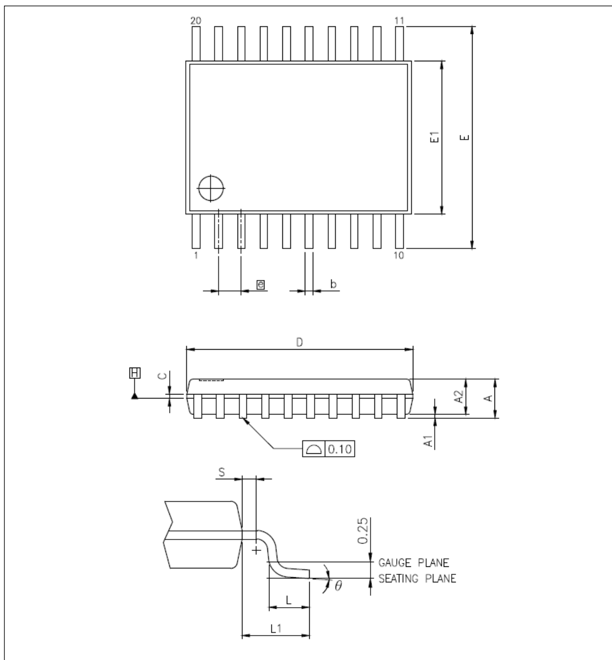
图 31. TSSOP20 – 6.5 x 4.4 mm 20 引脚纤薄紧缩小尺寸封装图
