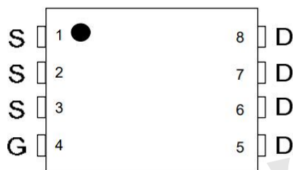
PDFN5X6-8
