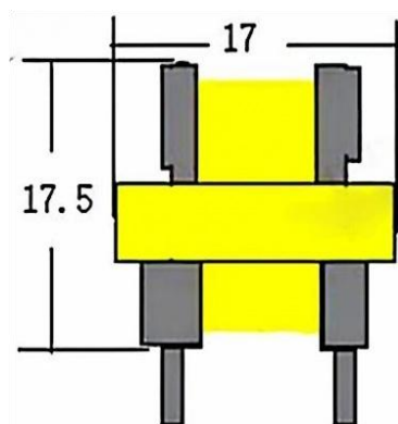
正视图
