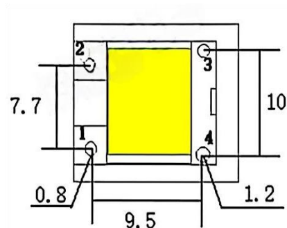
底视图
