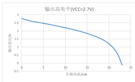
图 3 输出高电平与负载电流 ( V_{CC}=2.7\text{V} )
