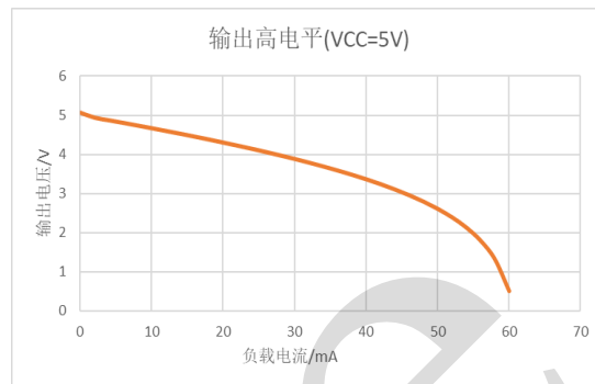
图 2 输出高电平与负载电流 ( V_{CC}=5\text{V} )
