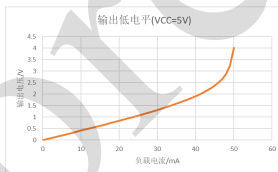
图 4 输出低电平与负载电流 ( V_{CC}=5\text{V} )
