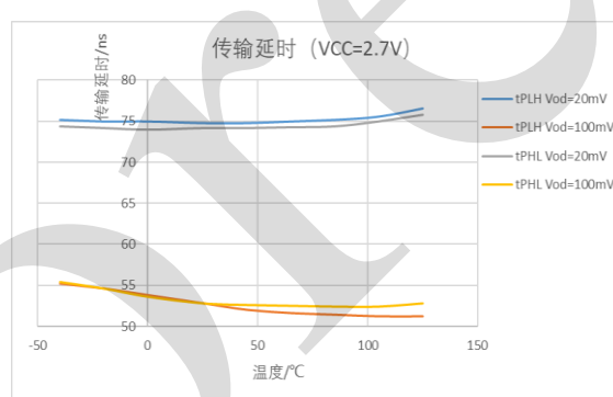
图 9 传输延时与温度 ( V_{CC}=2.7V )
