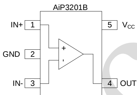
SOT553/SOT23-5
