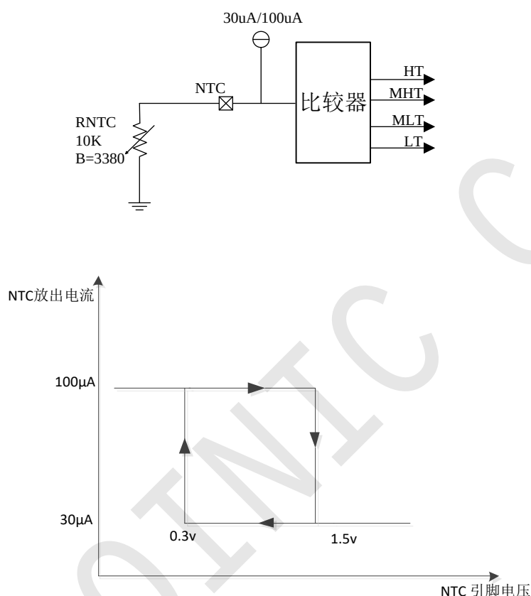
图 8 NTC 框图
