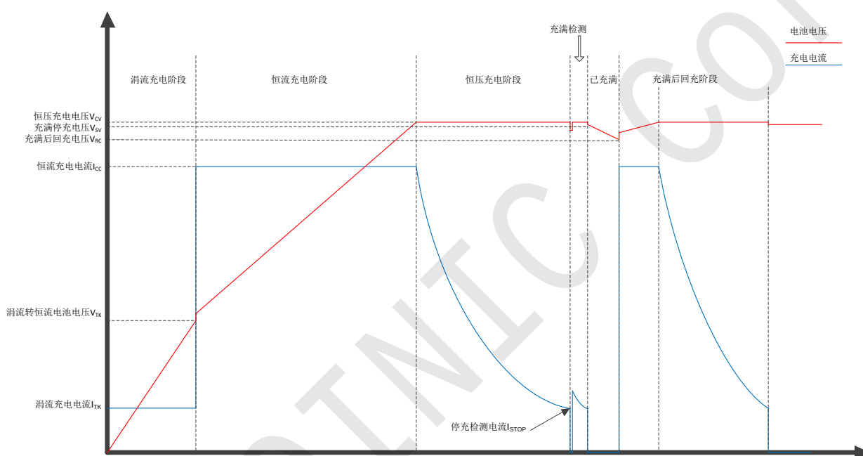
图 7 IP2332N 充电过程示意图
