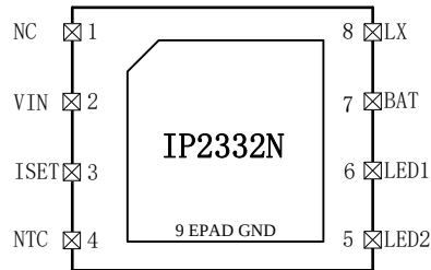
图 2 IP2332N 引脚图
