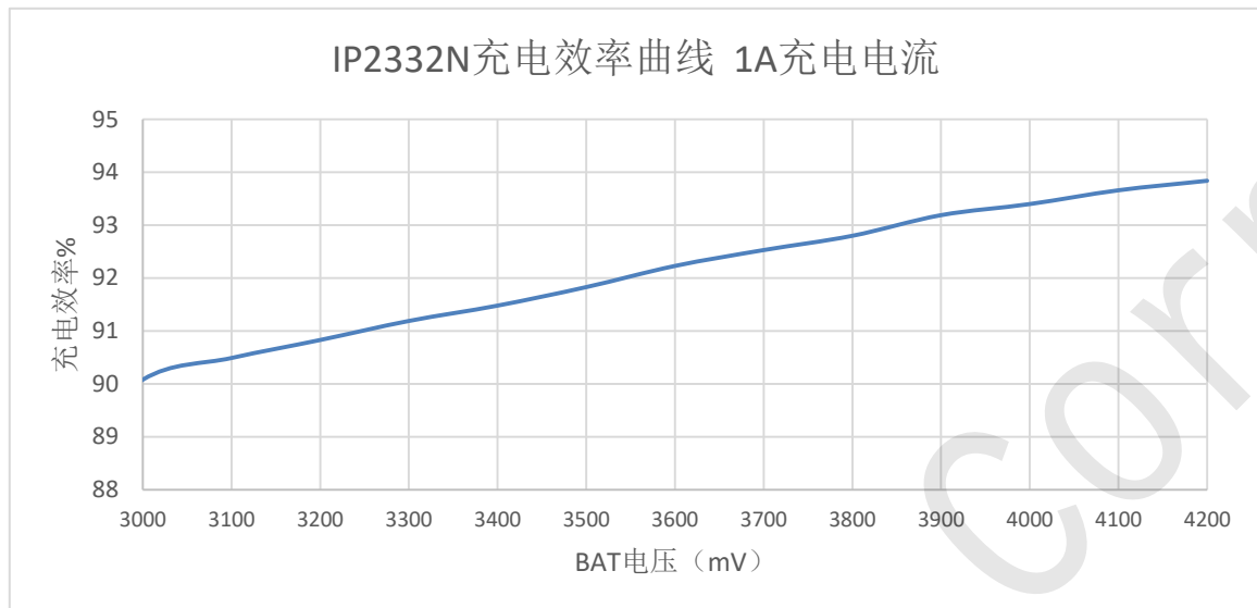
图 4 IP2332N 1A 充电效率曲线
