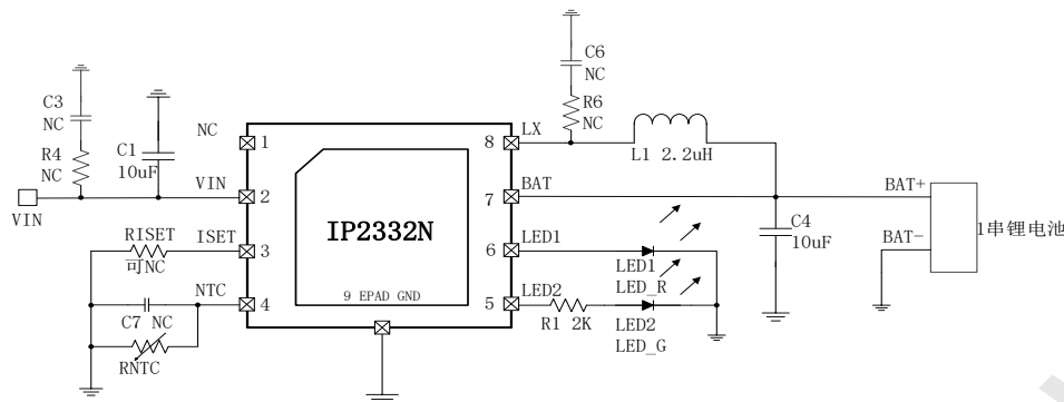
图 10 典型应用原理图
