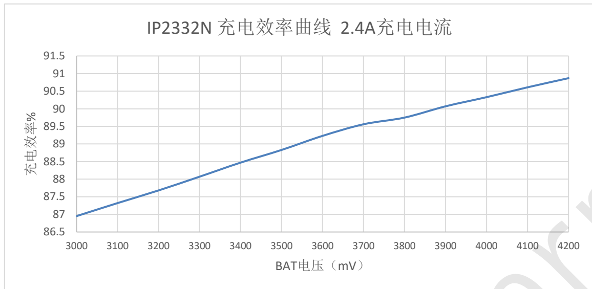
图 6 IP2332N 2.4A 充电效率曲线
