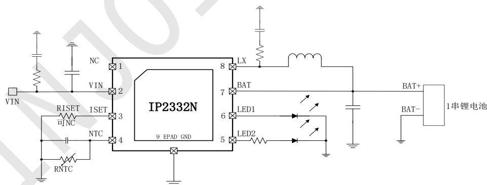
图 1 简化应用原理图
