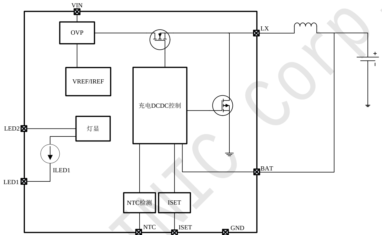
图3 IP2332N 内部框图
