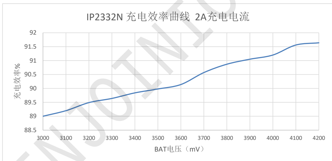
图 5 IP2332N 2A 充电效率曲线
