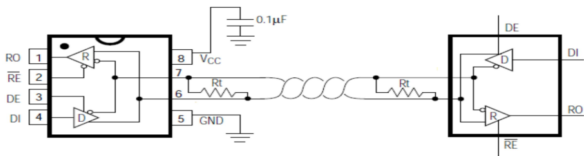
图 1： SP481EEN-TD典型半双工应用电路
