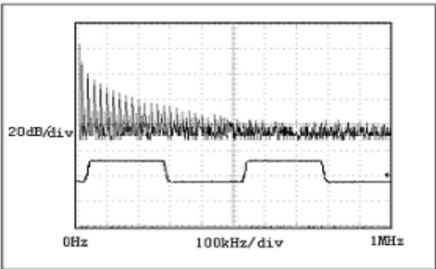
图11: 传输20kHz 信号时SP481EEN-TD驱动器输出波形和FFT图
