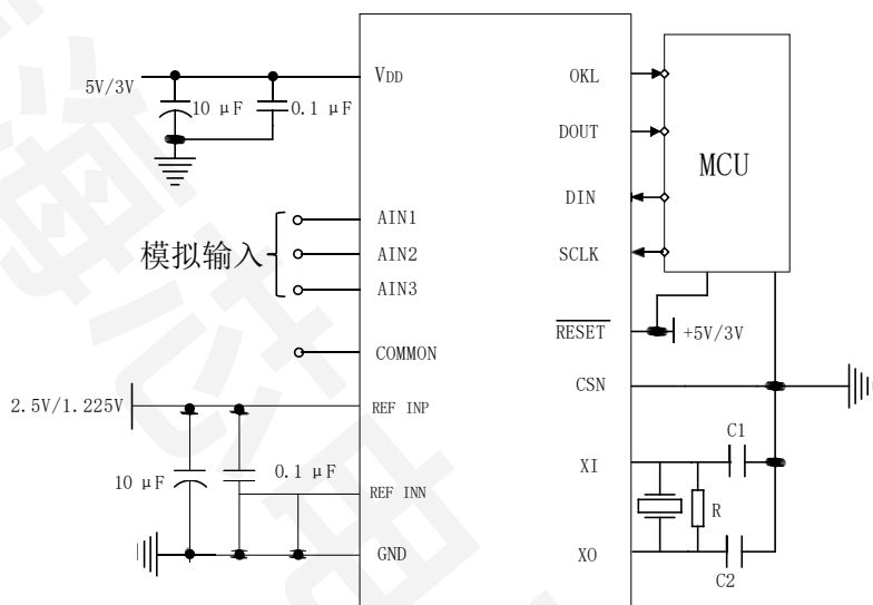
图 5 AD7706BNZ-HX/AD7706BRZ-HX/AD7706BRUZ-HX 的电路图
