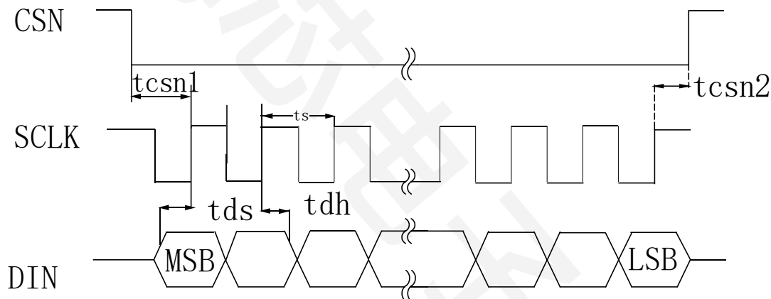
图 3 写时序
