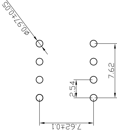
PCB开孔
