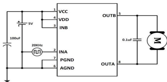
时间参数测试原理图
