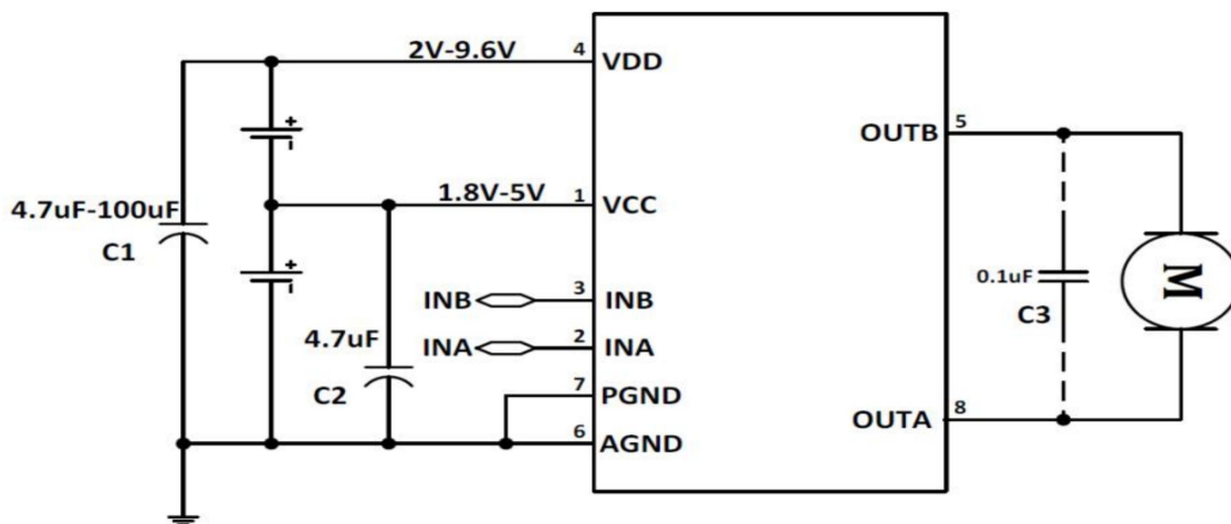
图 1 MX618-TD典型应用线路图
