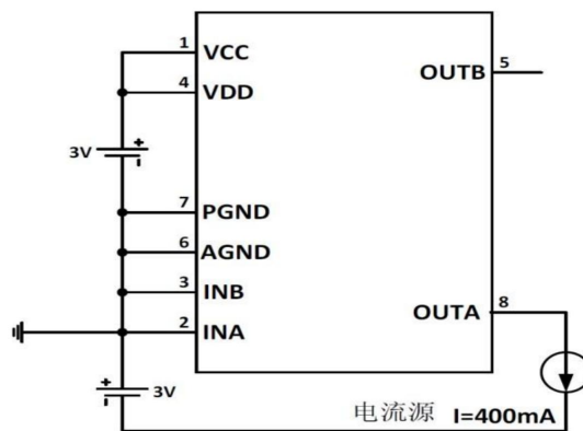
NMOS 体二极管导通电压测试原理图
