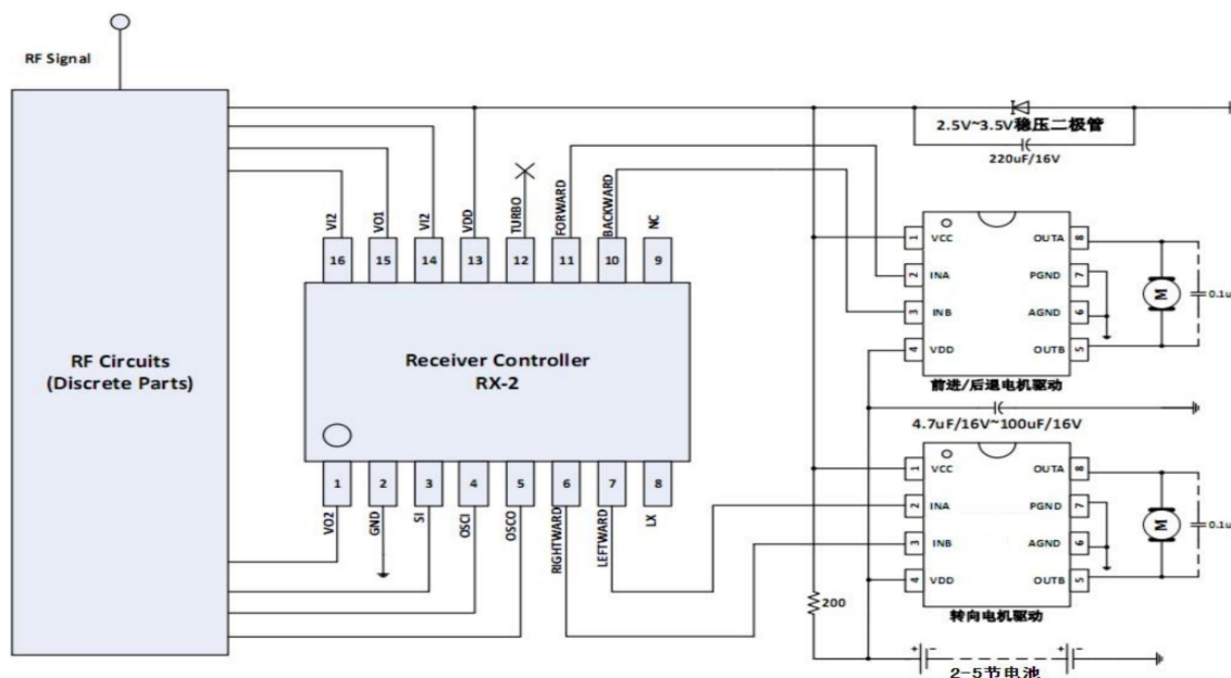
图 2 2-6 节电池供电玩具遥控车马达驱动应用线路图
