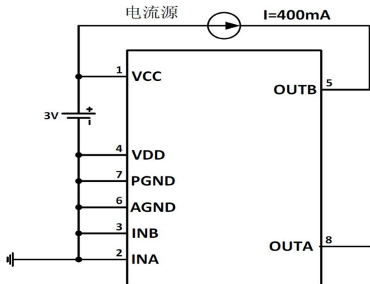
PMOS 体二极管导通电压测试原理图
