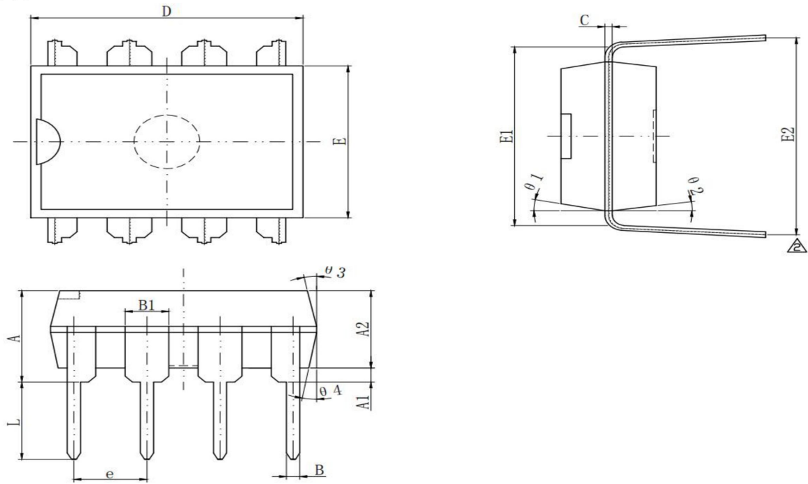
DIP8封装
