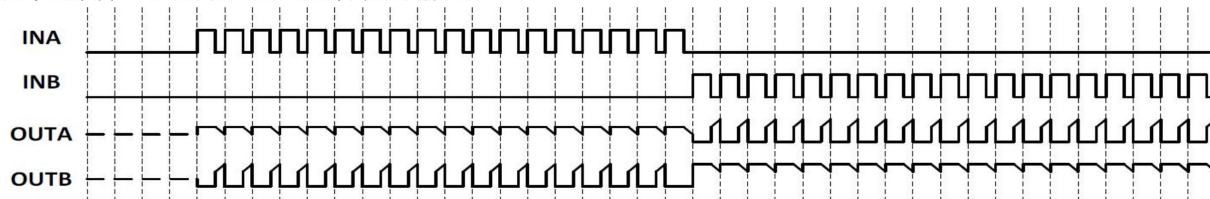
PWM模式A信号波形示意图
