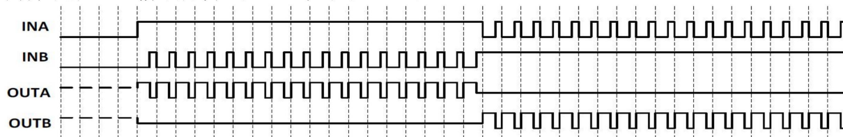
PWM模式B信号波形示意图
