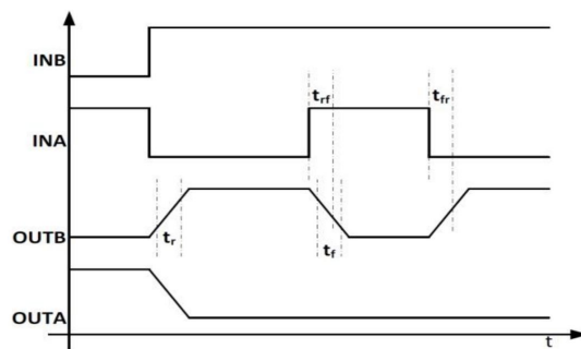
时间参数定义
