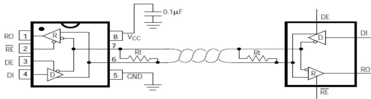
图 1： SP483EEN-TD典型半双工应用电路
