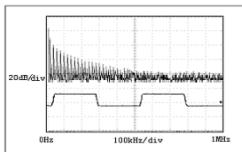
图11: 传输20kHz 信号时SP483EEN-TD驱动器输出波形和FFT图
