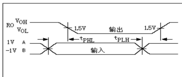
图 8:接收器传播延时
