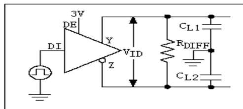
图 4:驱动器定时测试负载
