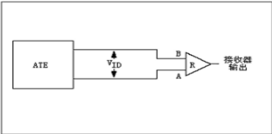
图 10:接收器传播延时测试电路
