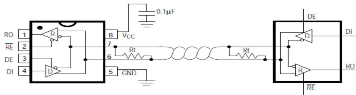
图 1： SP481ECN-TD典型半双工应用电路
