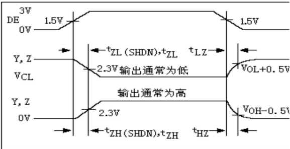
图 7:驱动器使能和无效时间
