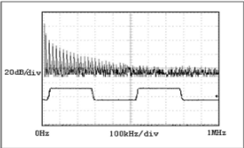
图11: 传输20kHz 信号时SP481ECN-TD驱动器输出波形和FFT图
